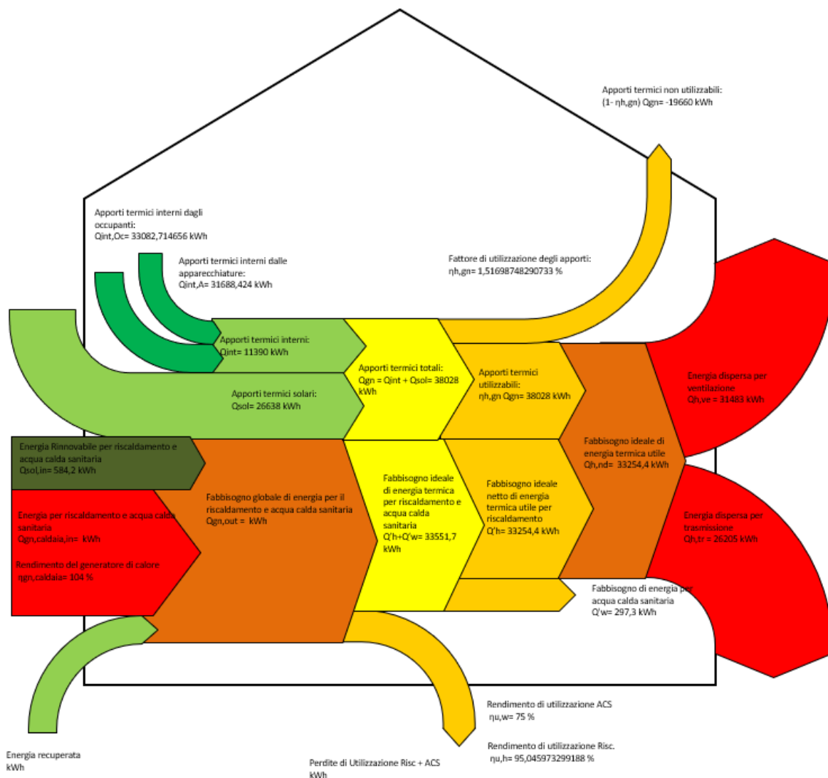
Figura 9.15 – SCN1: Diagramma di Sankey relativo al fabbisogno termico post intervento
