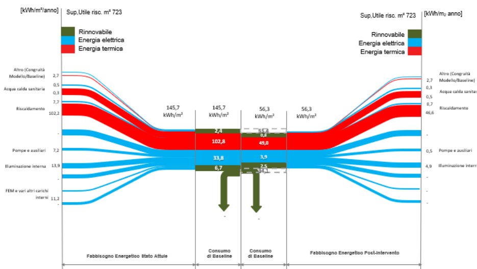
Figura 9.22 – SCN2: Bilancio energetico complessivo dell’edificio post intervento
