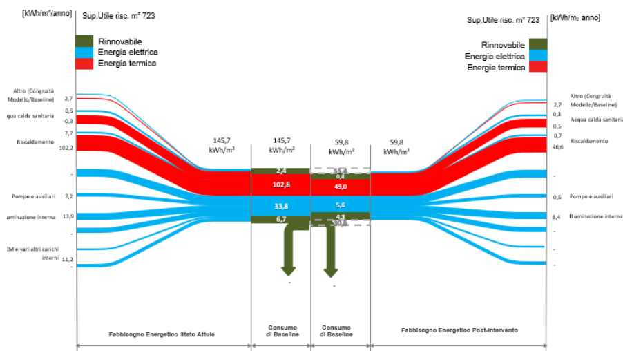
Figura 9.16 – SCN1: Bilancio energetico complessivo dell’edificio post intervento
