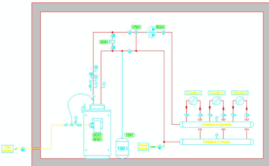
Figura 4.8 - Particolare dello schema di impianto
