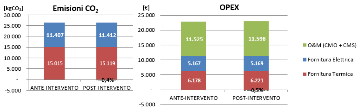
Figura 8.11 – EEM6: Riduzione dei costi operativi e delle emissioni di CO2 a partire dalla baseline
