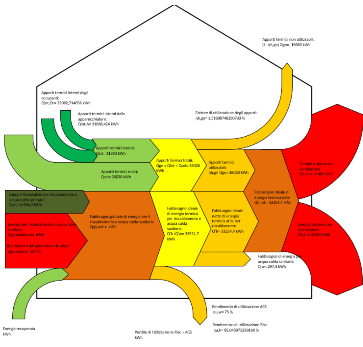
Figura 9.21 – SCN2: Diagramma di Sankey relativo al fabbisogno termico post intervento
