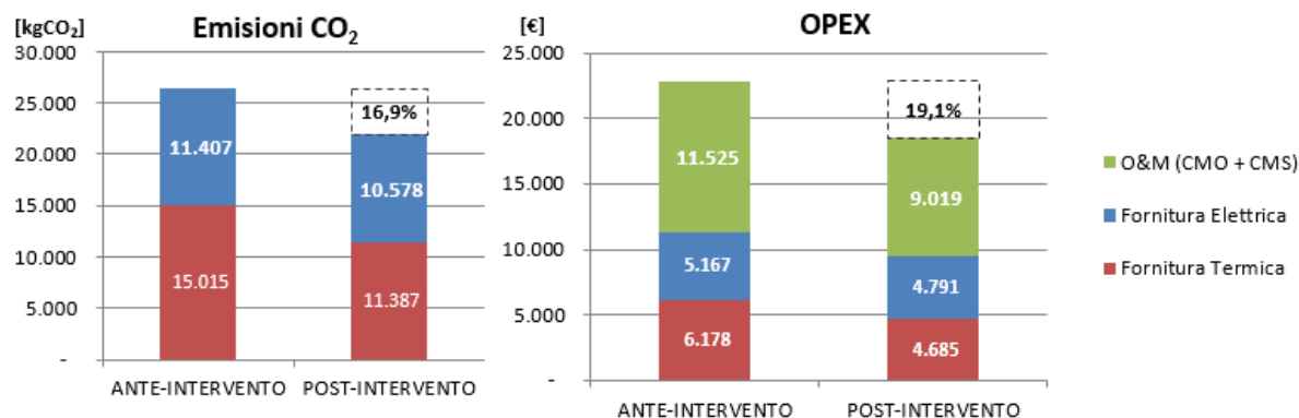
Figura 8.9 – EEM7: Riduzione dei costi operativi e delle emissioni di CO 2 a partire dalla baseline
