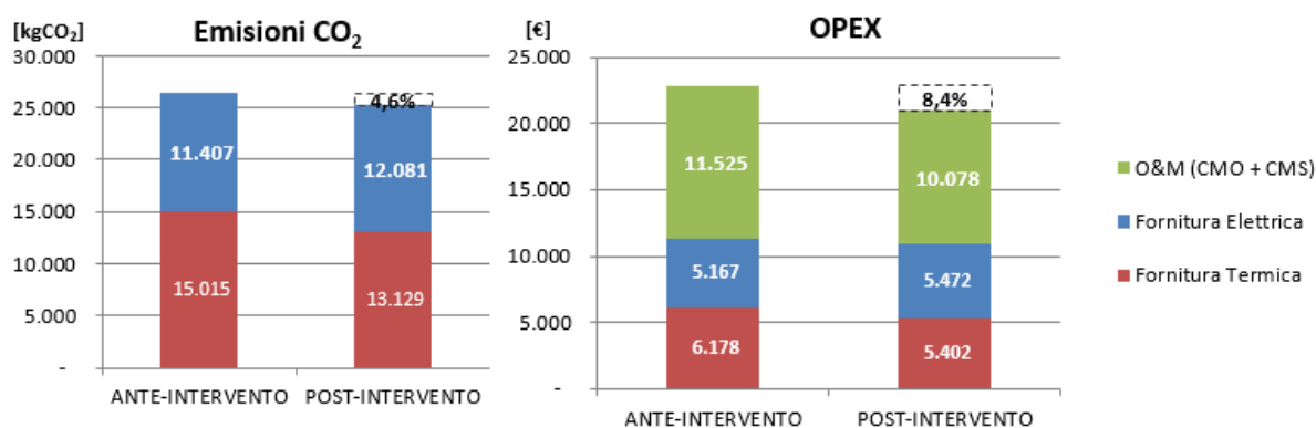
Figura 8.7 – EEM5: Riduzione dei costi operativi e delle emissioni di CO2 a partire dalla baseline
